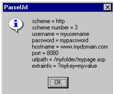
Figure -1: ParseUrl の出力
