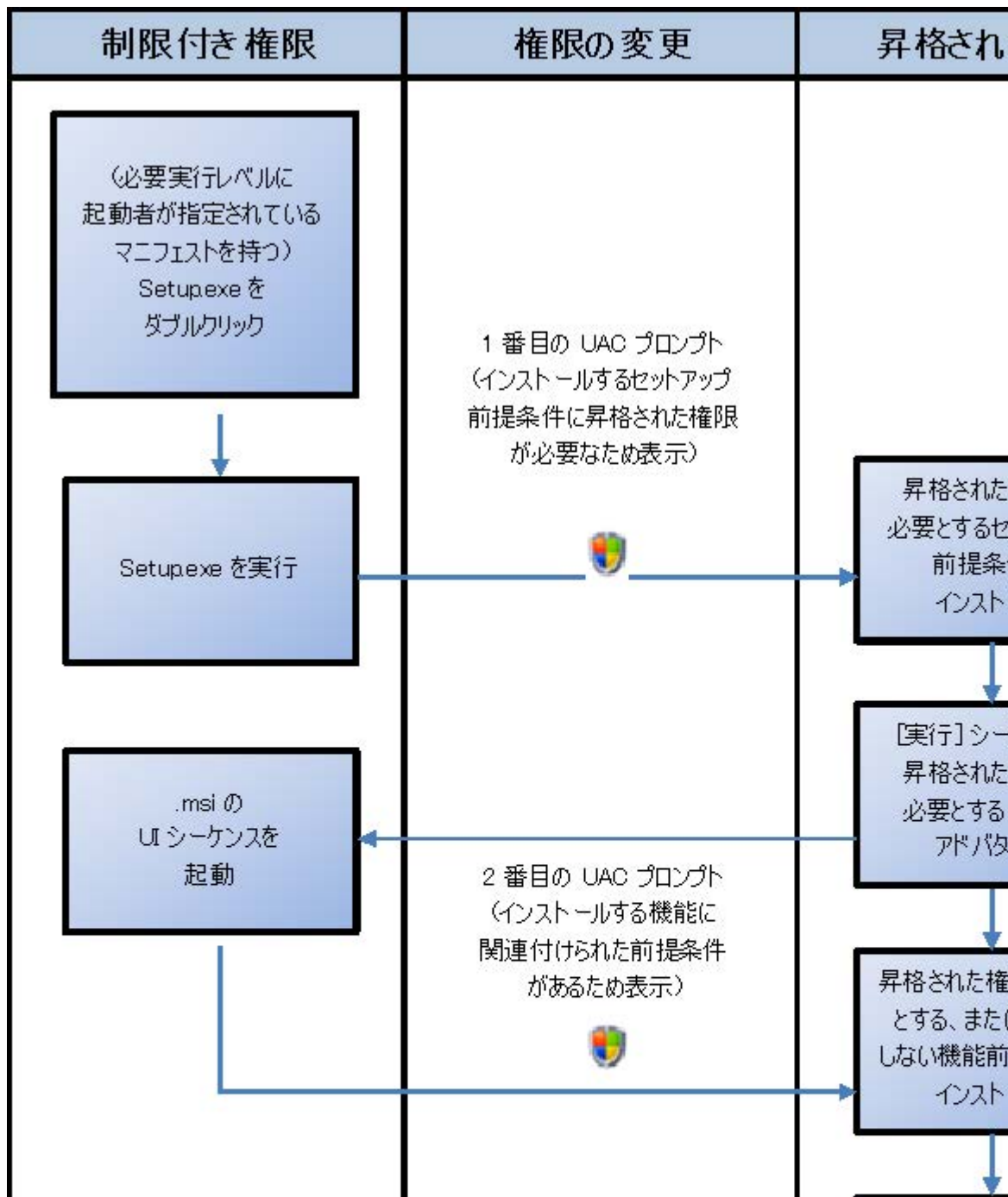
図 1: 例 1: “必要実行レベル” が [起動者] で、かつ .msi ファイルをアドパタイズするインストールのダイアグラム
